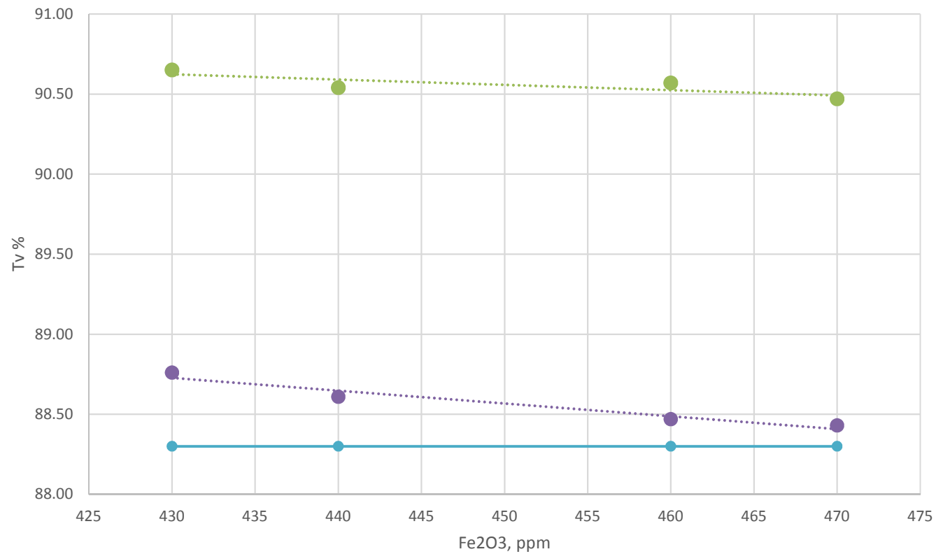
FÉNYÁTERESZTÉS - ÜVEG VASOXID-TARTALMA
